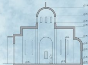
ПРЕСЕК Б-Б P=1:100
