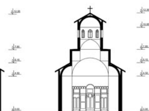
ПРЕСЕК 2-2 Р=1:100
