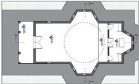
ОСНОВА ПРИЗЕМЉА Р 1:100
