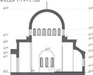
ПРЕСЕК 1-1 Р=1:100
