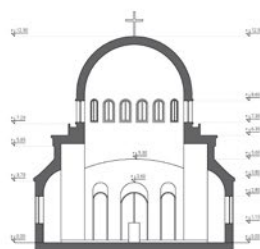
ПРЕСЕК 2-2 Р=1:100
