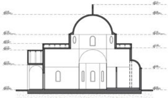
ПОДУЖНИ ПРЕСЕК Р 1:100
