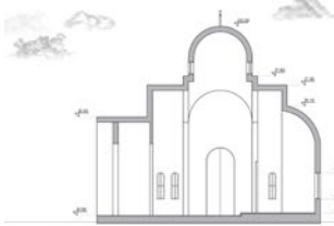
ПОДУЖНИ ПРЕСЕК P=1:100
