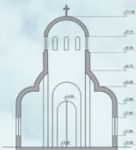
ПРЕСЕК А-А P=1:100
