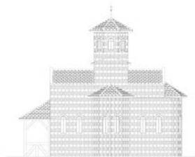
ЈУЖНА ФАСАДА Р=1:100
