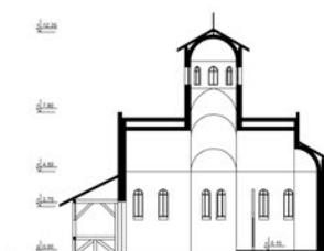
ПРЕСЕК 1-1 Р=1:100
