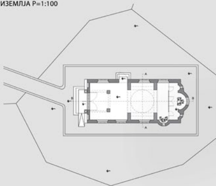
ОСНОВА ПРИЗЕМЛЈА Р=1:100
