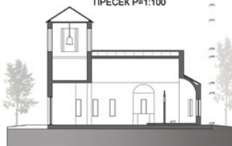
ПОДУЖНИ ПРЕСЕК P=1:100
