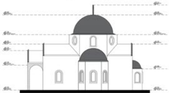
ИЗГЛЕД ЈУЖНЕ ФАСАДЕ Р 1:100
