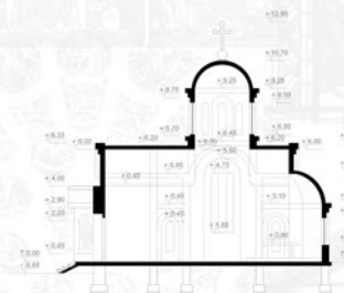
ПОДУЖНИ ПРЕСЕК Р=1:100
