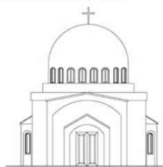
ЗАПАДНА ФАСАДА Р=1:100
