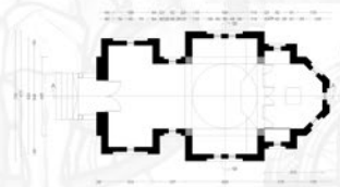
ОСНОВА ПРИЗЕМЉА Р=1:100
