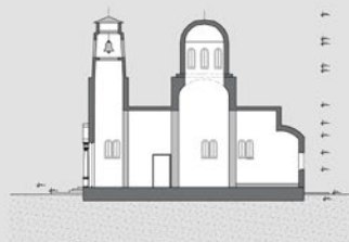
ПОДУЖНИ ПРЕСЕК Р=1:100
